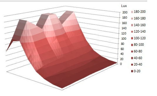
مخطط (5) مخطط ثلاثي الأبعاد لمستويات الإضاءة الناتجة من استخدام 3 انابيب ضوئية بقطر 36سم. المصدر : الباحثان
