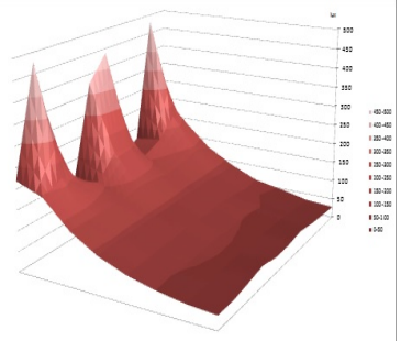
مخطط (1) مخطط ثلاثي الأبعاد لمستويات الإضاءة الناتجة من الشبائيك ضمن التوجيه الشمالي. المصدر : الباحثان
