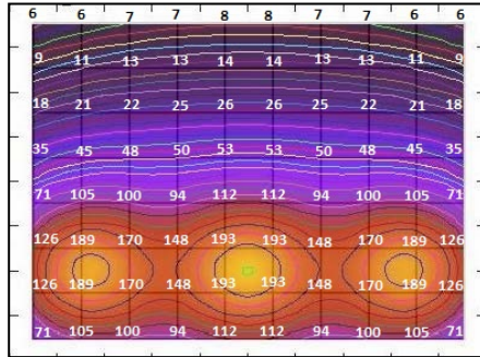
شكل (17) مستويات الإضاءة الداخلية ل3 انابيب في برنامج (Holigilm) لكل متر ضمن التوجيه الشمالي. المصدر : الباحثان
