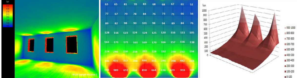
شكل (16ب) منظور داخلي للقاعة يوضح الحد الأعلى والادنى لمستويات الإضاءة السنوية للواجهة الجنوبية. المصدر : الباحثان
